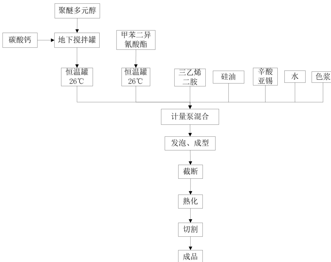
图 2-4 汽车用海绵生产工艺流程图
