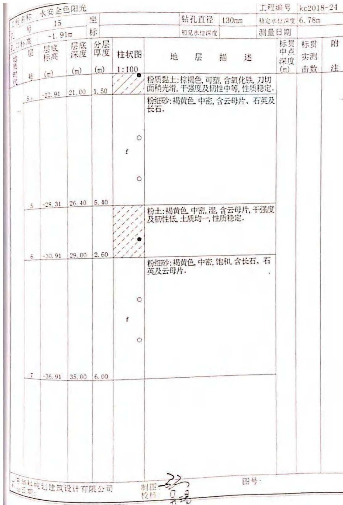
图2.1-5 钻孔柱状图 (部分)
