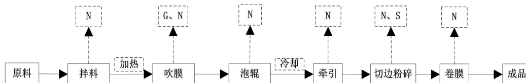
图 2-4 本项目生产工艺流程及产污环节图
