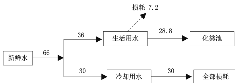
图 2-3 项目水平衡图 (m³/a)
