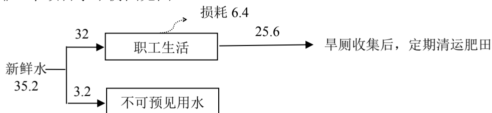
图 2-3 本项目水平衡图 (m³/a)
